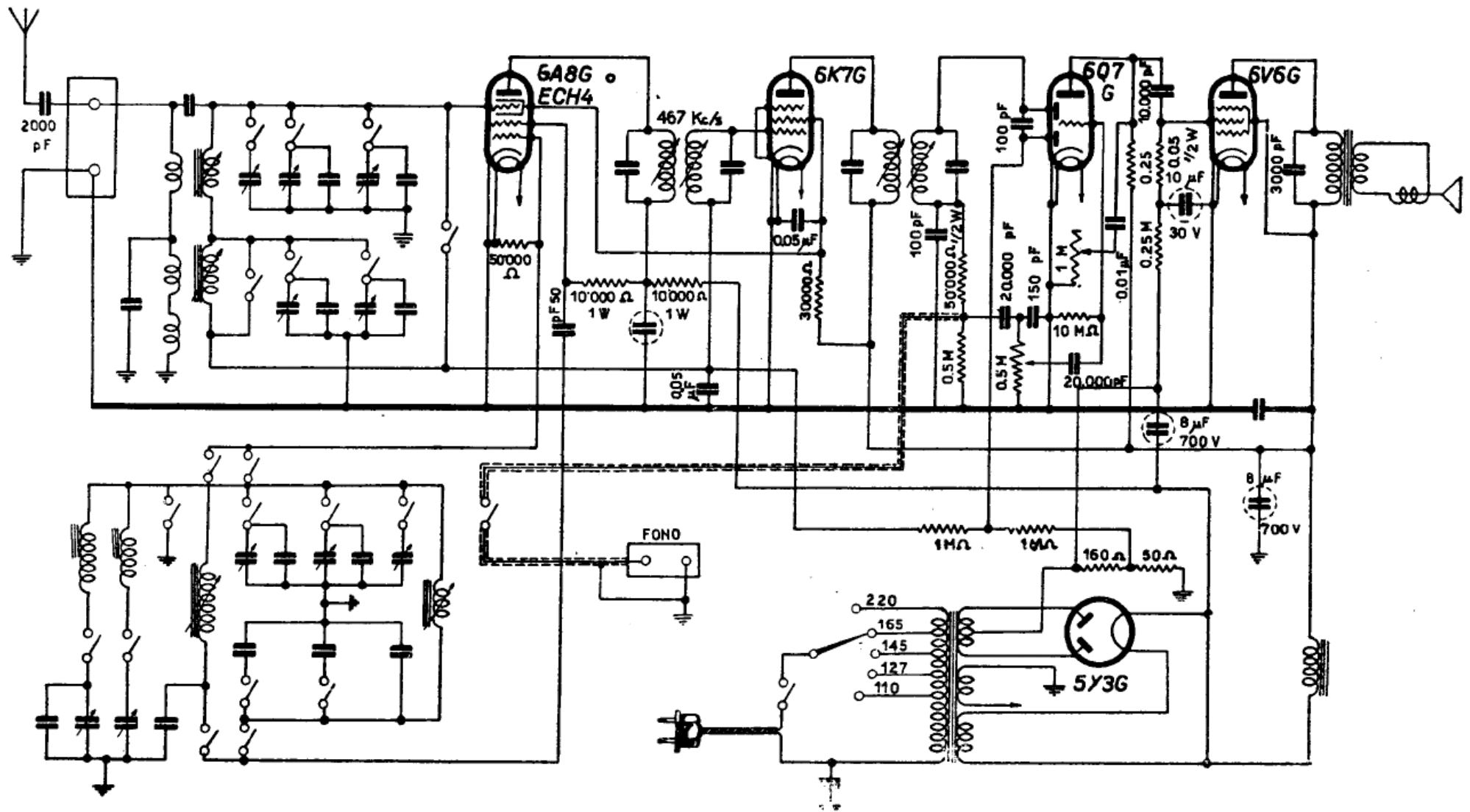
ELECTA RADIO - Mod. ER 46 - Supereterodina con sintonia a permeabilità. Media frequenza: 467 kc/s. Potenza: 4 W circa. Sensibilità: 40 \mu V circa. Consumo: 60 W circa. Produzione 1946.
